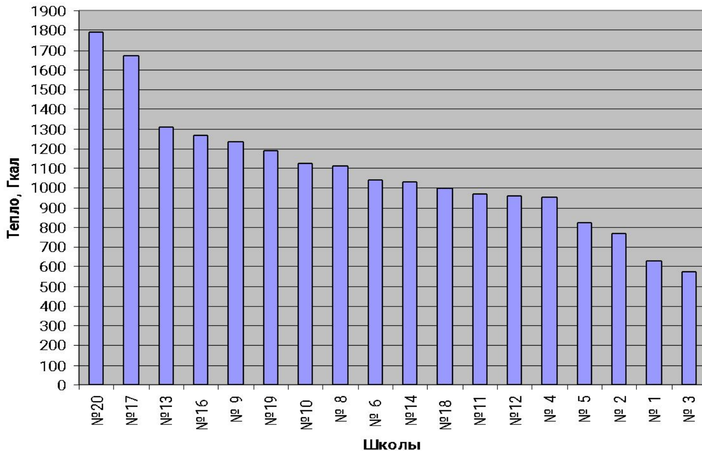
Потребление тепла в школах г. Новочебоксарск за 2009 г.
