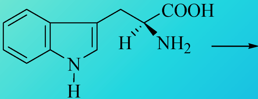
триптофан
