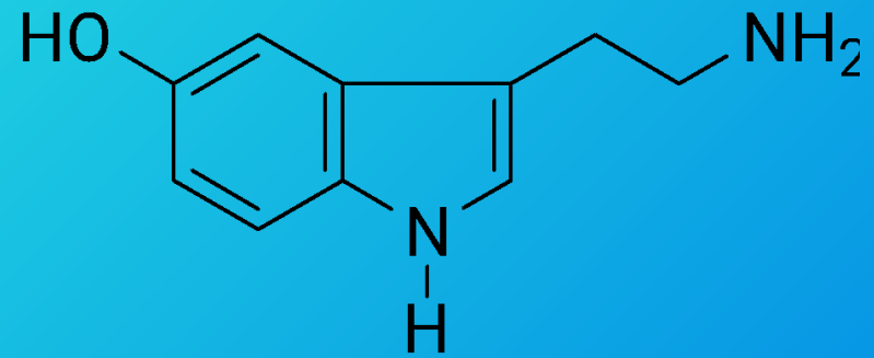
серотонин
