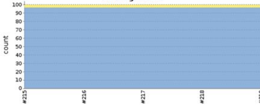
FindBugs Trend
