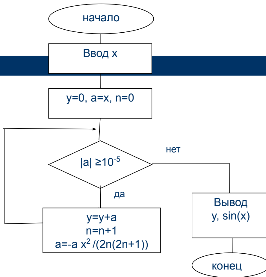
Рис. 2.1. Схема алгоритма вычисления y = \sin x
