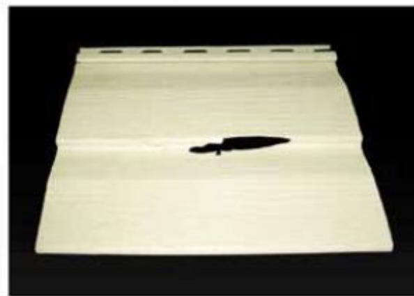
Фото 10. Образец сайдинга одного из российских производителей после проведения теста №2.
