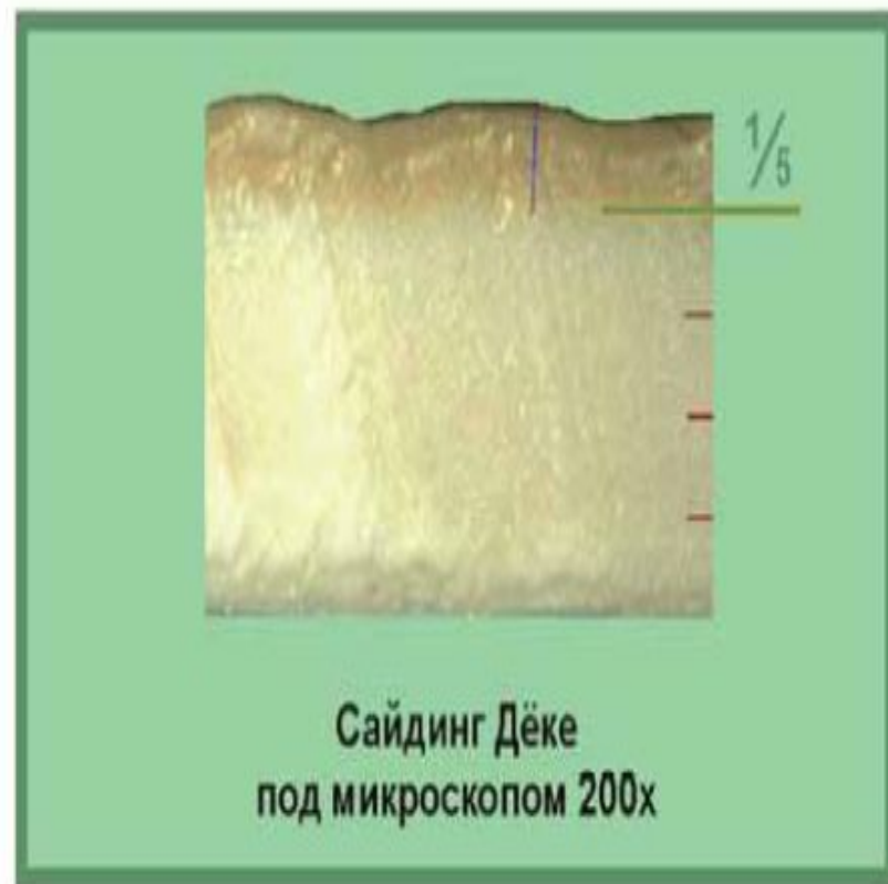
Пример 3. Сайдинг Дёке под микроскопом 200х.
