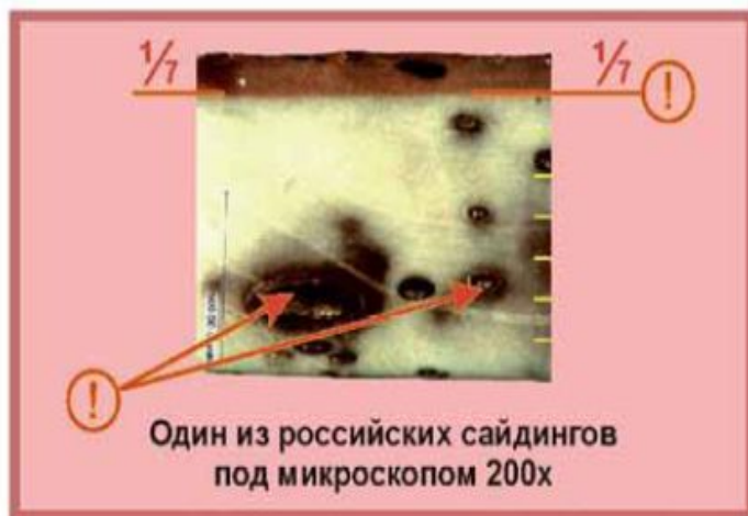
Пример 2. Один из российских сайдингов под микроскопом 200х.
