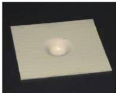
Фото 4. Результат теста ASTM для сайдинга Дёке при превышении ударных усилий на 50%.
