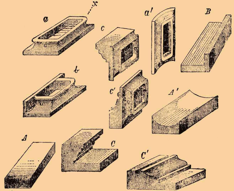
а, а', б, в, с, с'—печные изразцы для разных частей печи. А, А', В, С, С'—формы или коладки, при помощи которых изготовляются изразцы.
