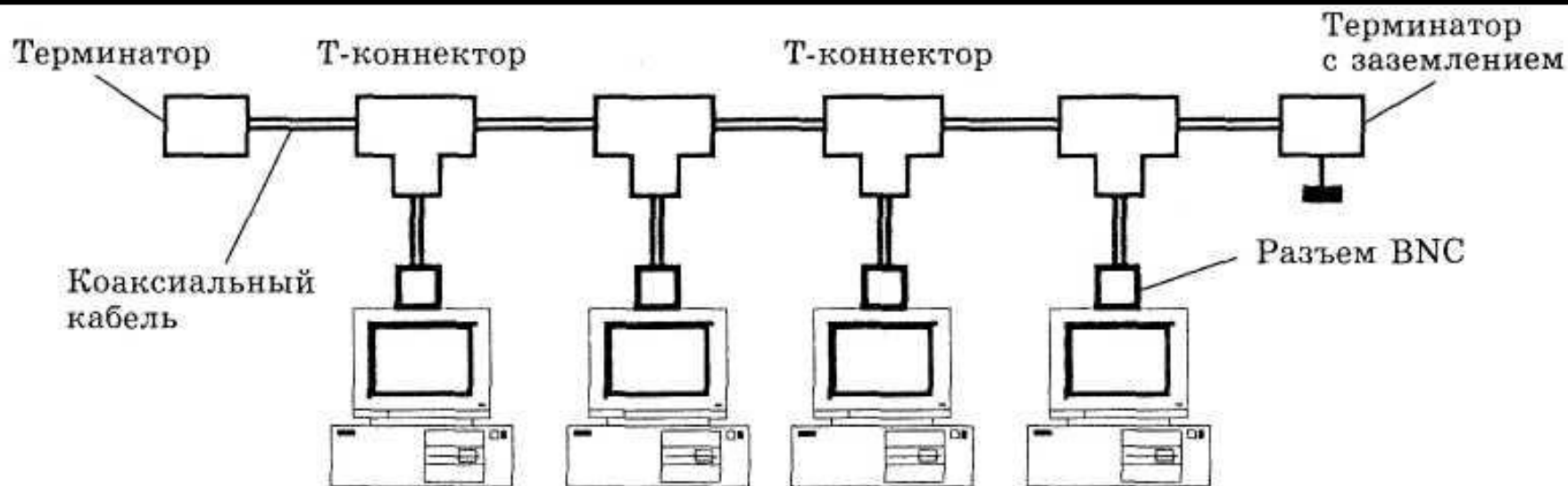
Рис. 1. ЛКС на тонком коаксиальном кабеле
