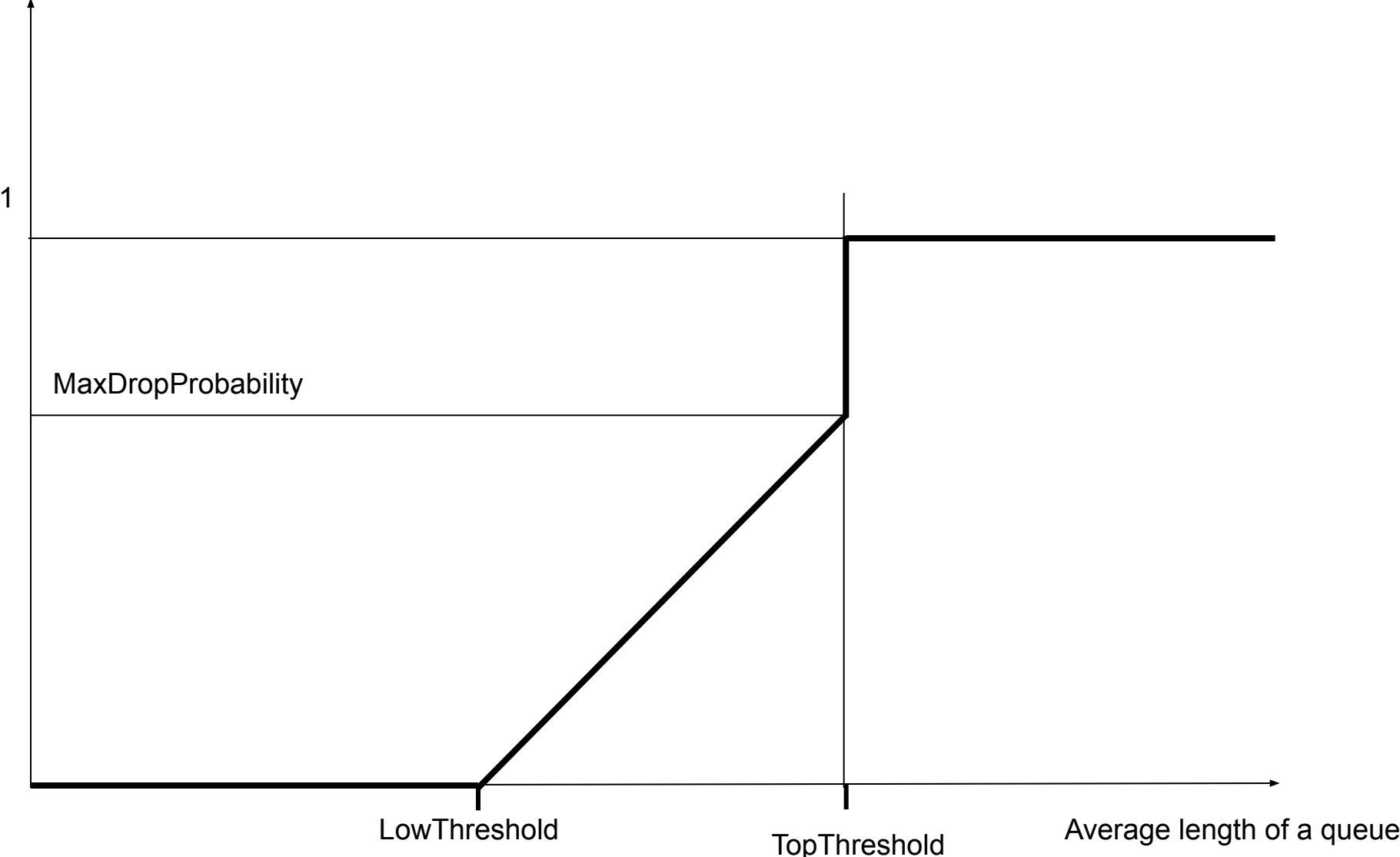
Рис. 20.2. Вероятность отбрасывания пакетов алгоритмом RED
