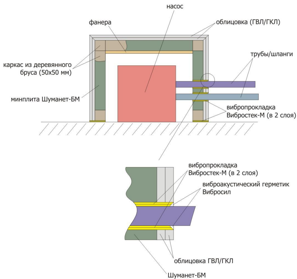
Схема звукоизоляции насоса
