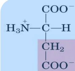
Aspartate
