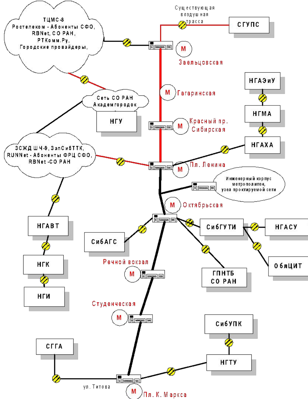
Схема ВОЛС образовательной сети Новосибирска по линии метрополитена
