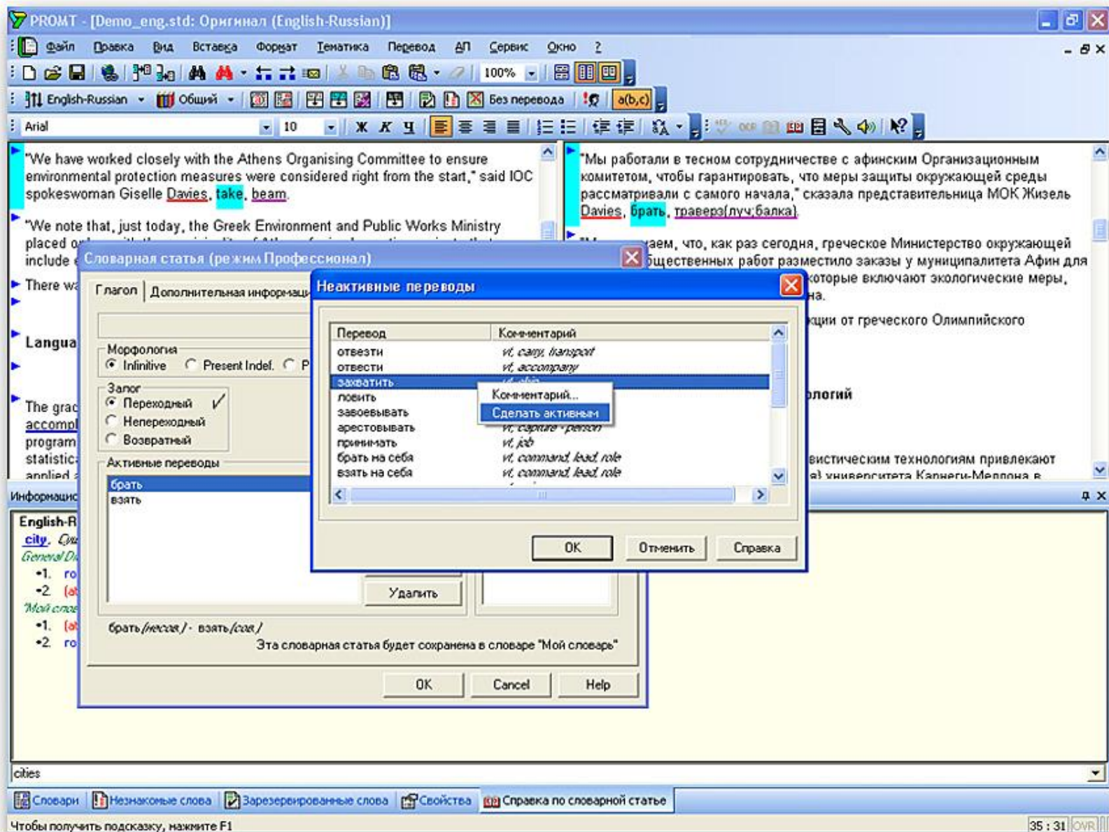
Рис 1. Процедура работы с активными и неактивными переводами.
