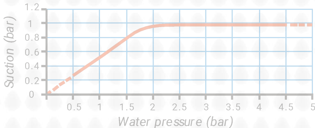
Производительность трубки Вентури
