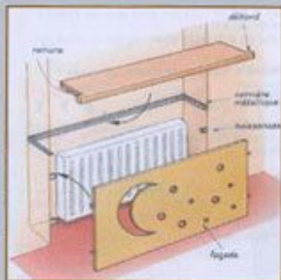
СХЕМА КРЕПЛЕНИЯ РАДИАТОРНОГО ПРОСТРАНСТВА
