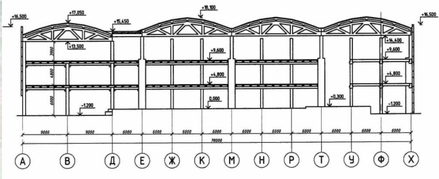
Разрез 1-1
