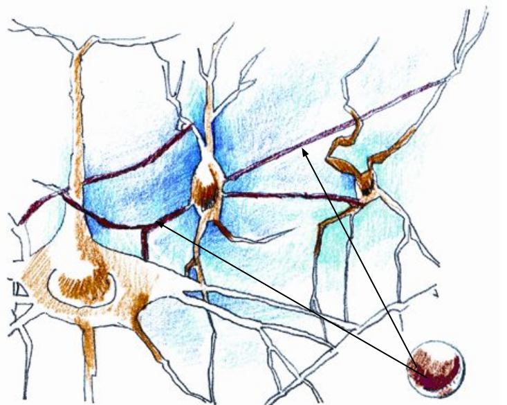
Метионин
