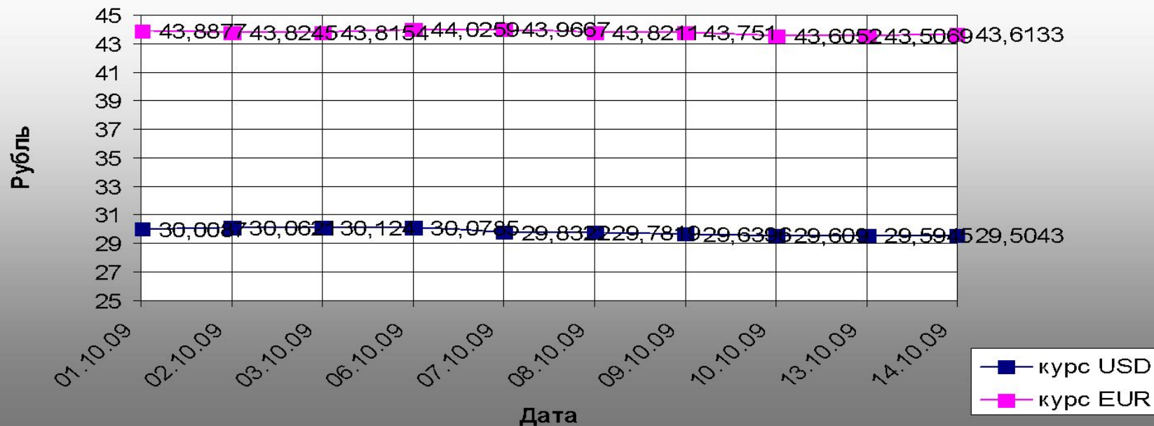
Курсы валют
