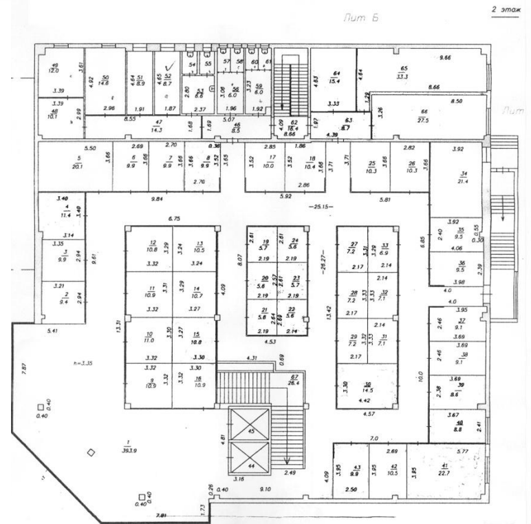
2 этаж
