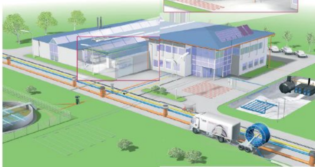
Системы теплоснабжения
