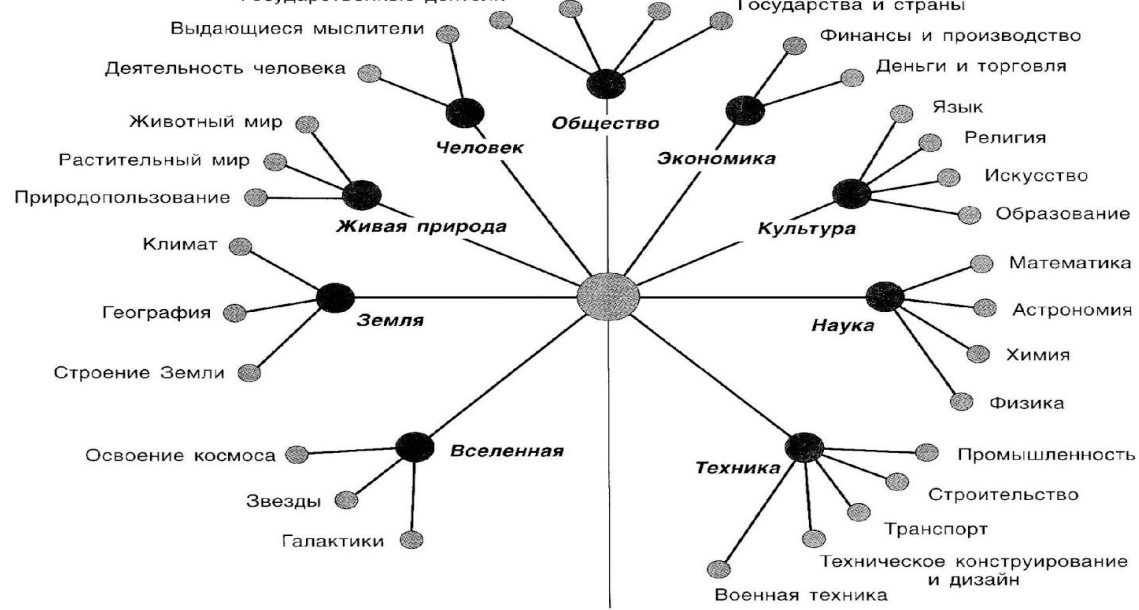
Рис. 3. Классификационное дерево
