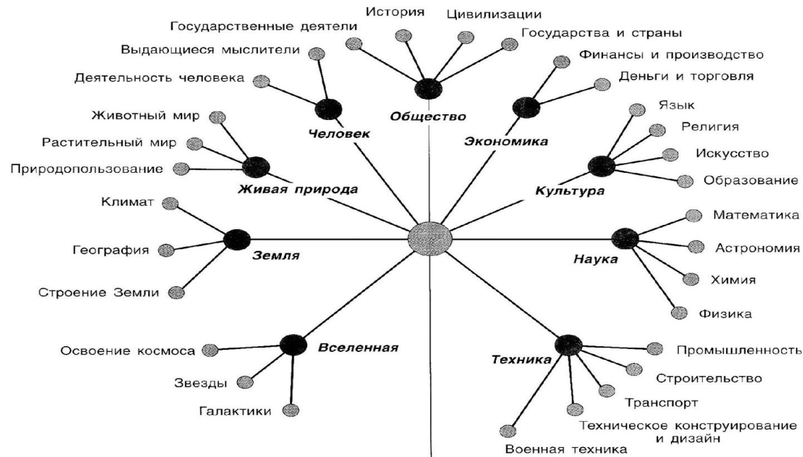
Рис. 3. Классификационное дерево
