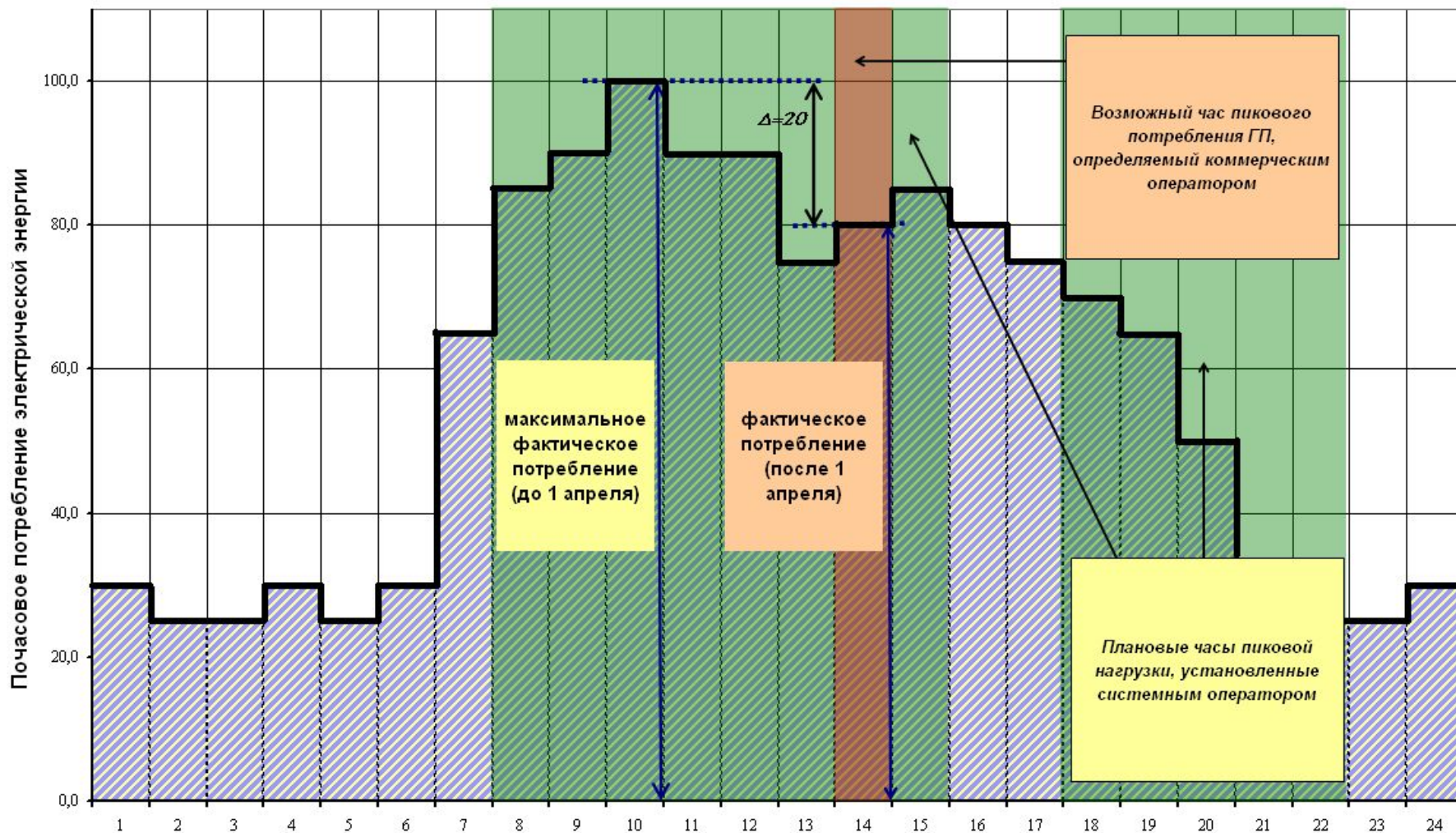
Суточный график нагрузки потребителя
