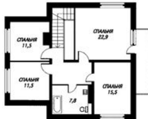
план 2 этажа
