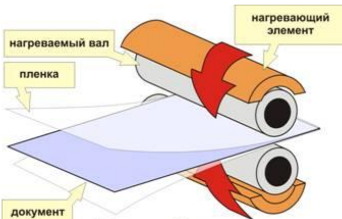
Схема работы ламинатора по технологии нагреваемых валов Модели: Photo ID, EXL A4 и EXL A3
