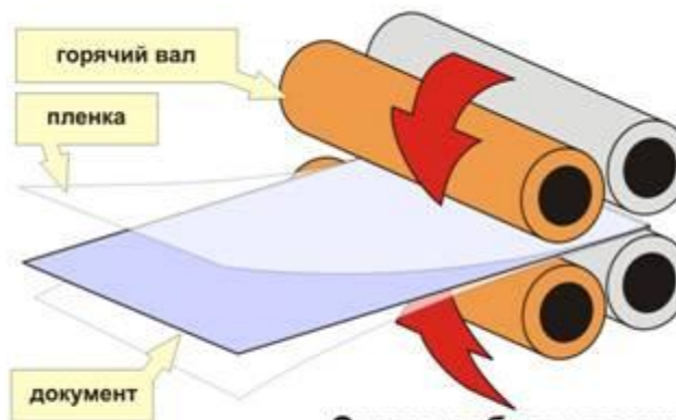
Схема работы ламинатора по технологии горячих валов Модели: HRLA4, HRLA3, SPLA4, SPLA3 и SPLA2
