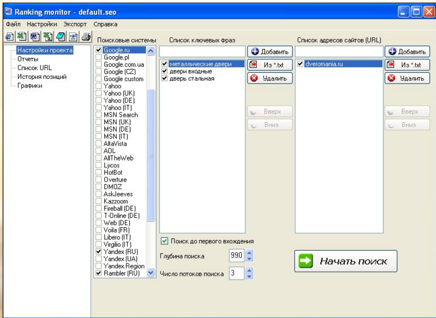
Панель настроек модуля проверки позиций программы Semonitor
