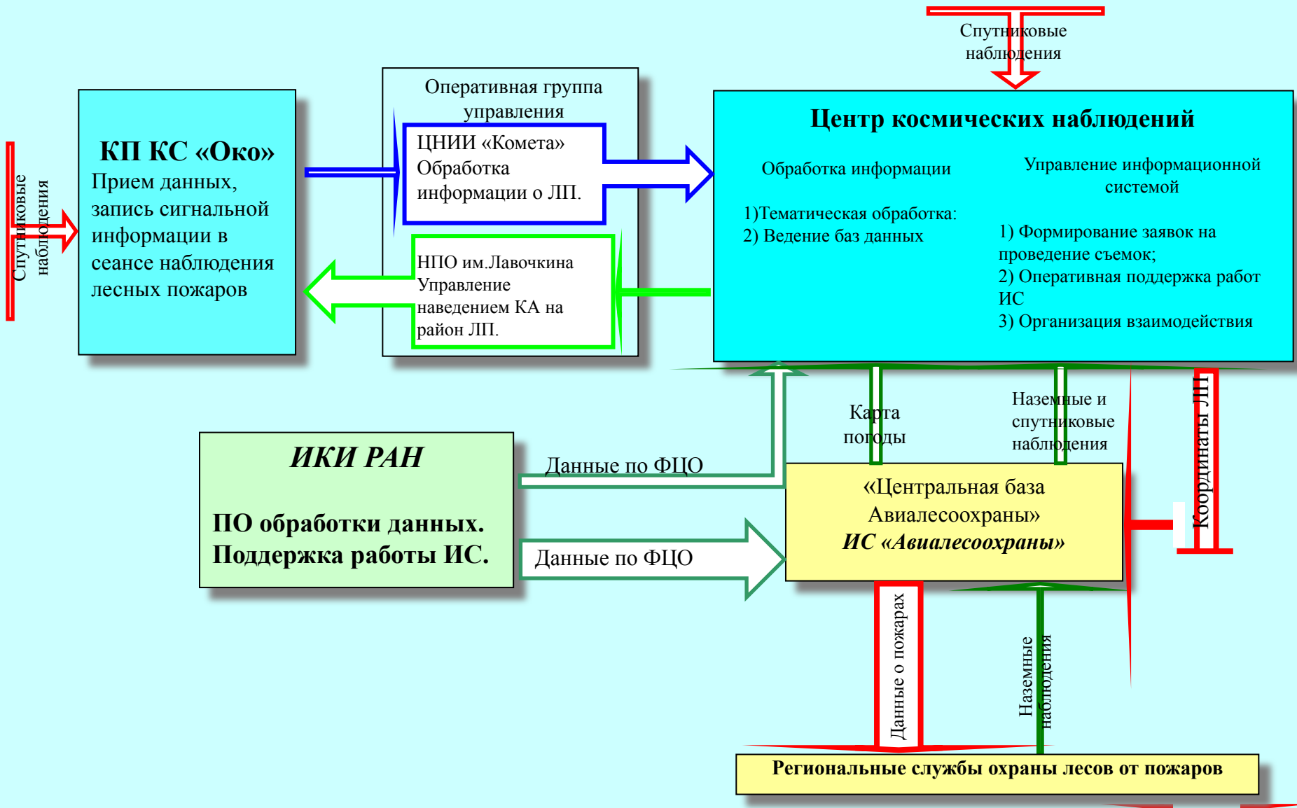
Схема проведения космического эксперимента по обнаружению лесных пожаров с КА на стационарной орбите
