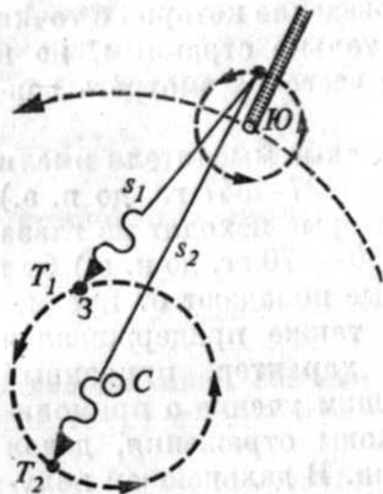
Рисунок 5.1. К определению скорости света Рёмером:
