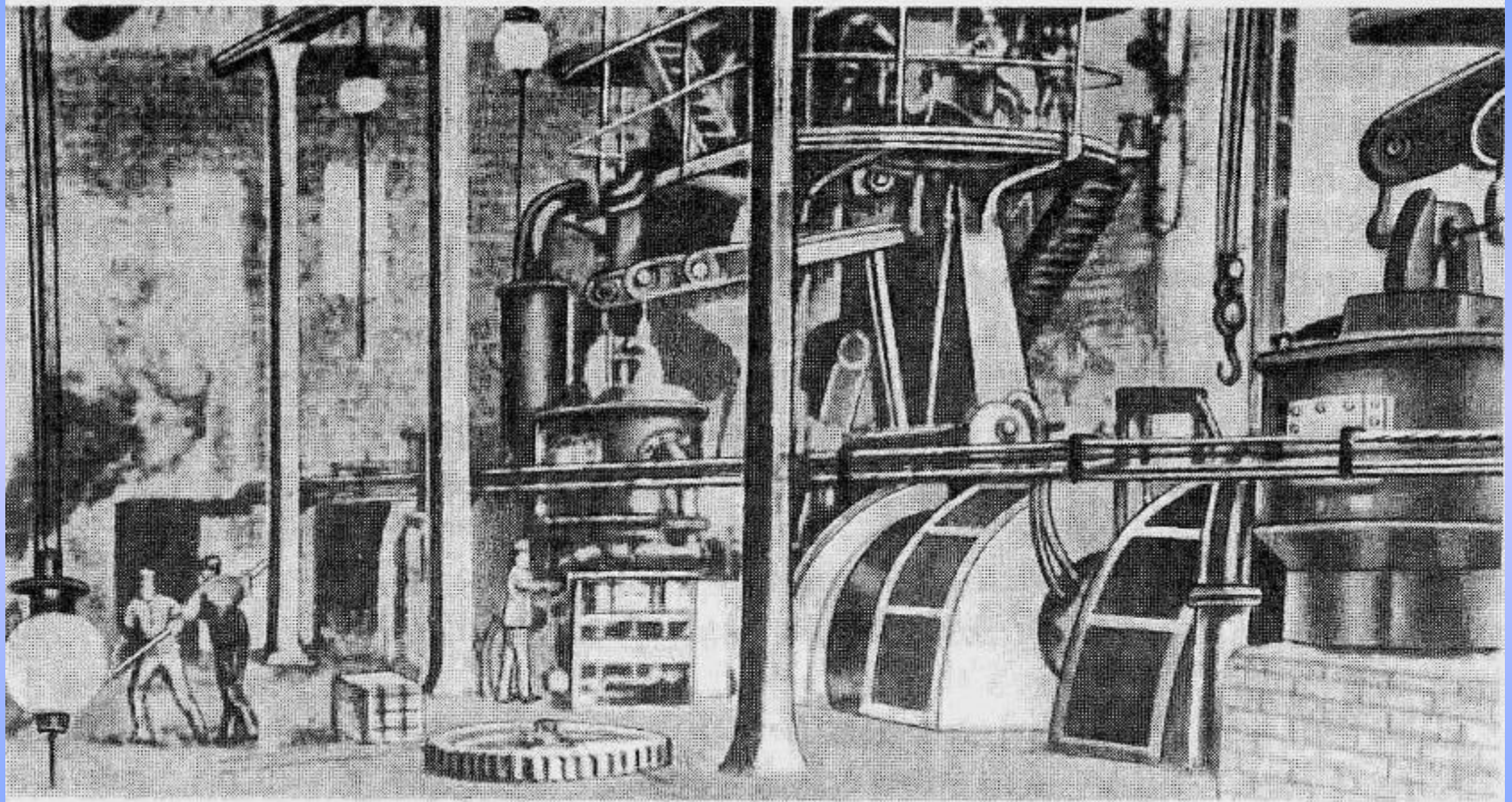
Машинный зал центральной электростанции в Берлине. 1890 г.
