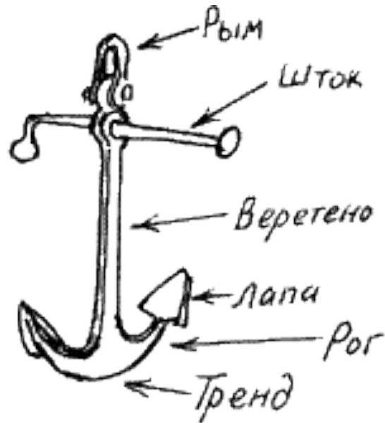
Современный адмиралтейский якорь
