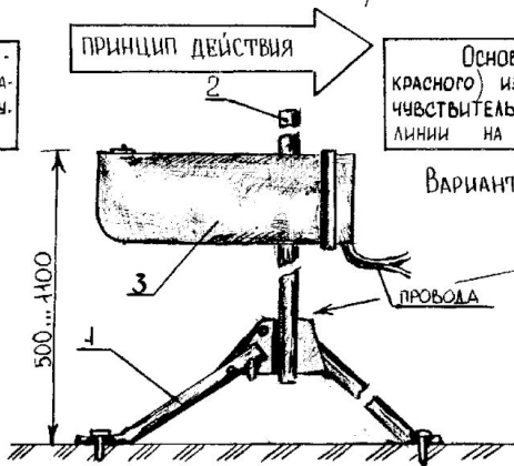
РИС. 1 Датчик. 1-стойка; 2-щтырь; 3-приёмник.
