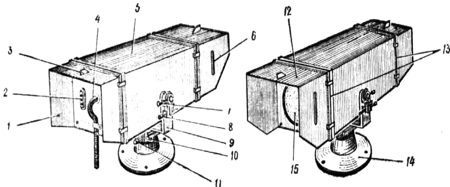
Рис. 3. Внешний вид устройств датчика обнаружения "МАК":
