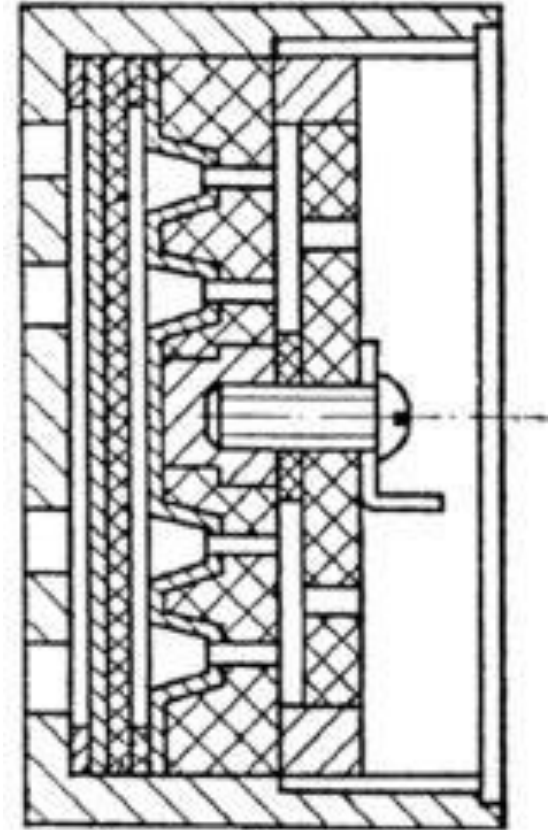
Конструкция капсулы конденсаторного микрофона
