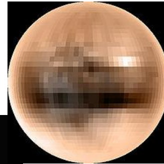
Плутон
