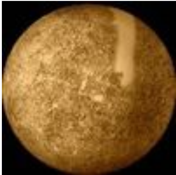
Меркурий
