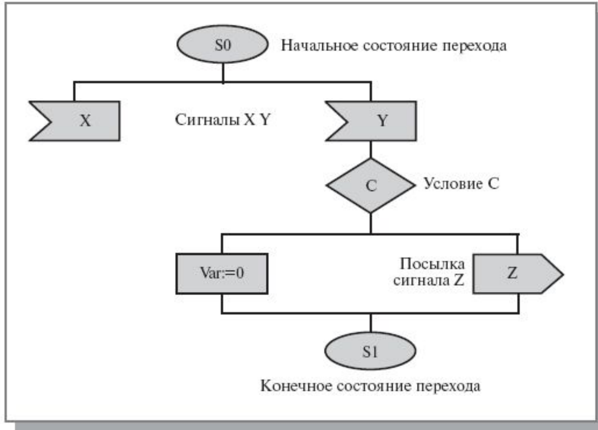
Пример SDL-диаграммы
