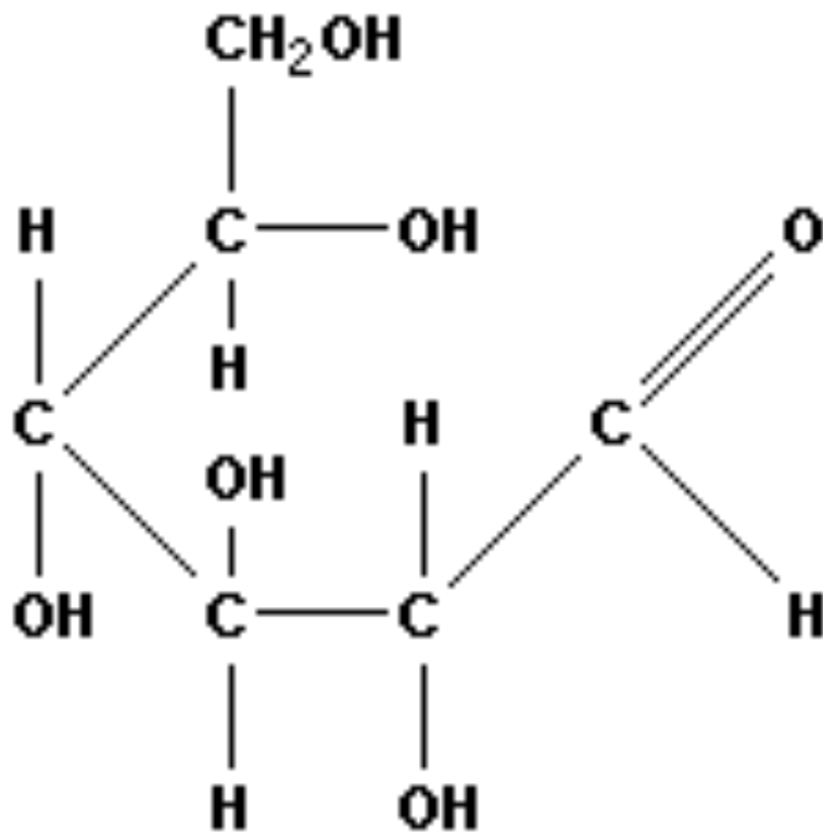
глюкоза (моносахарид)
