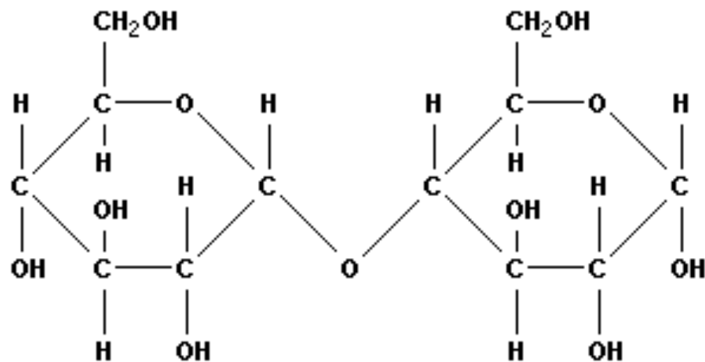
Мальтоза
