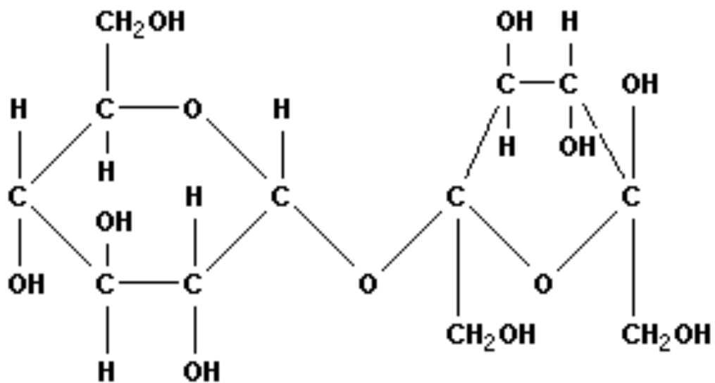
Сахароза
