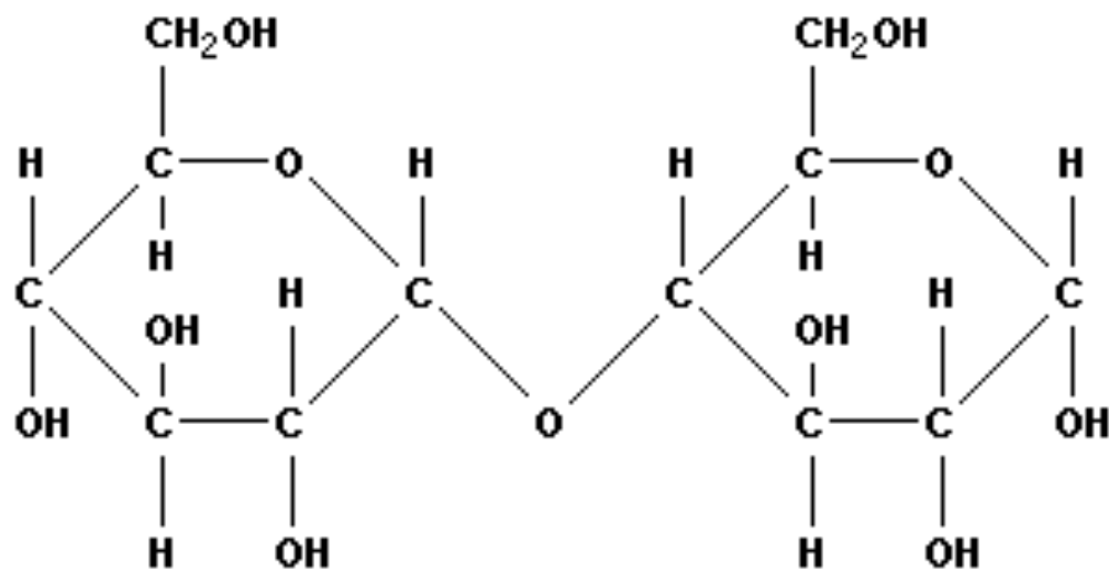
Мальтоза
