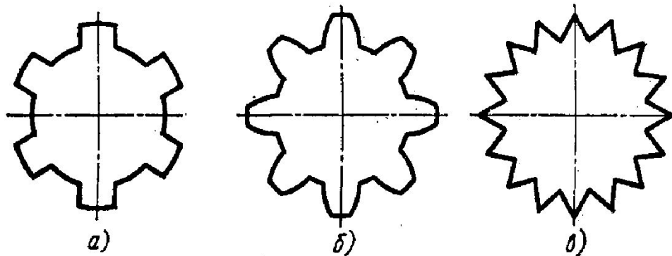
ВИДЫ ШЛИЦОВ
