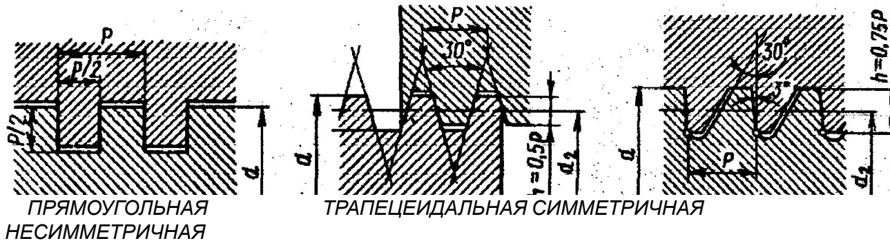
РЕЗЬБЫ ХОДОВЫЕ
