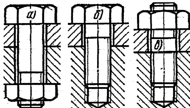
РЕЗЬБОВЫЕ СОЕДИНЕНИЯ
