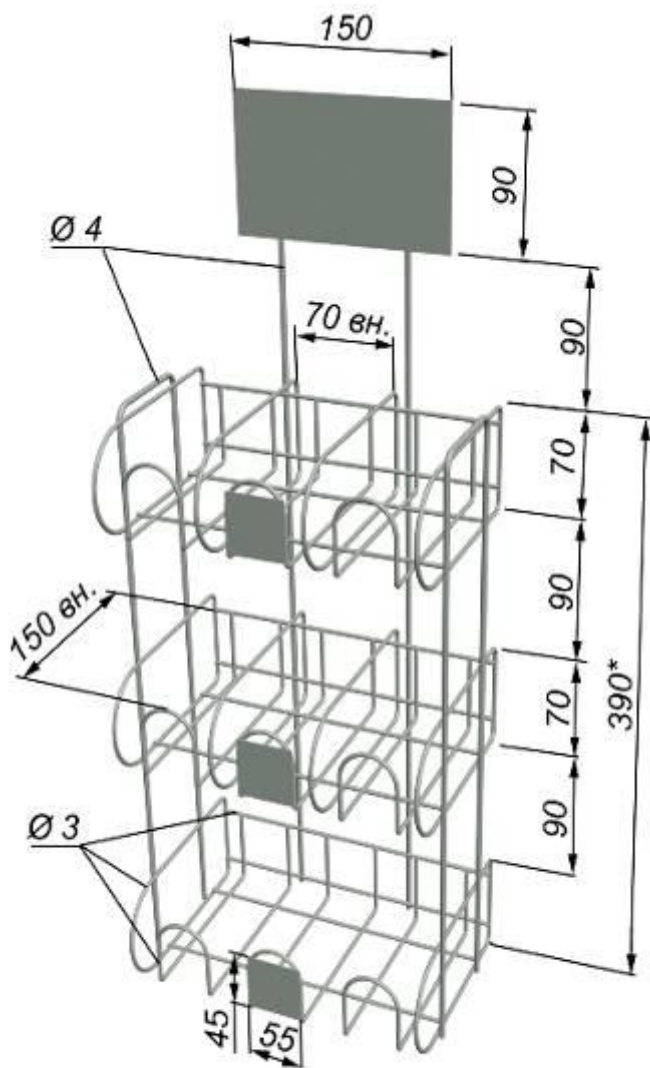
Дисплей "Хербалис 9"
