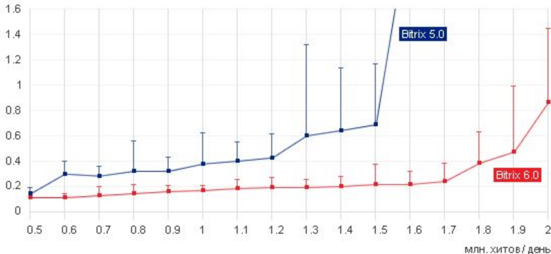
График «Время загрузки главной страницы, в зависимости от количества хитов в сутки (сек)»
