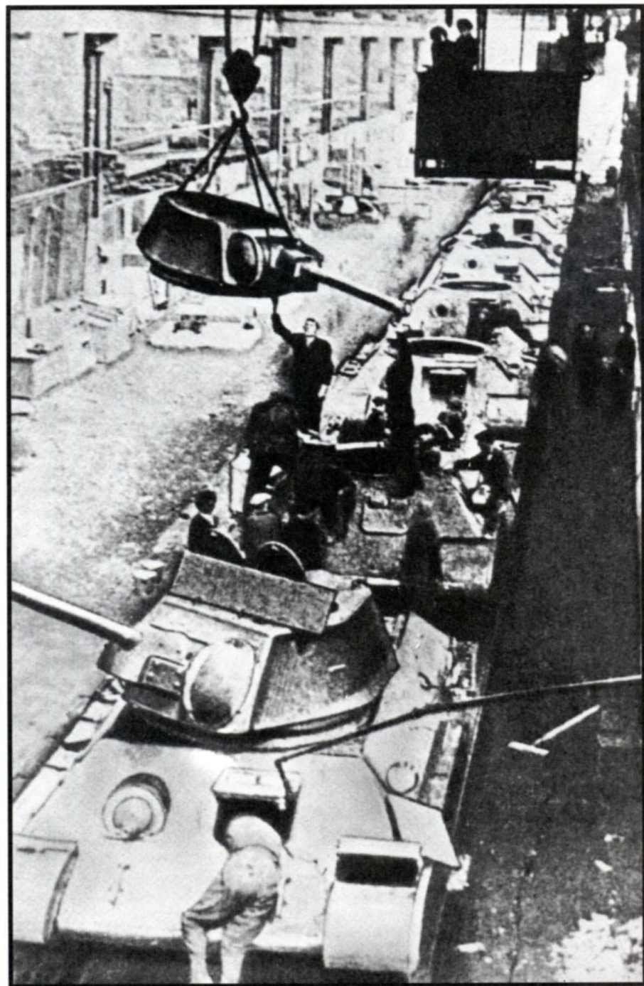
Сборка танков на Кировском заводе в Челябинске
