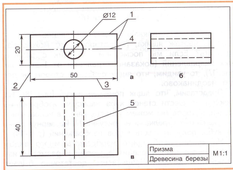
Рис. 2. Чертеж детали: а – главный вид; б – вид слева; в – вид сверху. Линии: 1 – контура, сплошная основная; 2 – выносная, сплошная тонкая; 3 – размерная, сплошная тонкая; 4 – осевая симметрии, штрихпунктирная; 5 – пунктирная невидимого контура
