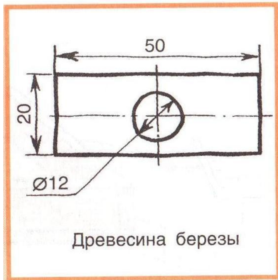
Рис. 3 . Эскиз детали
