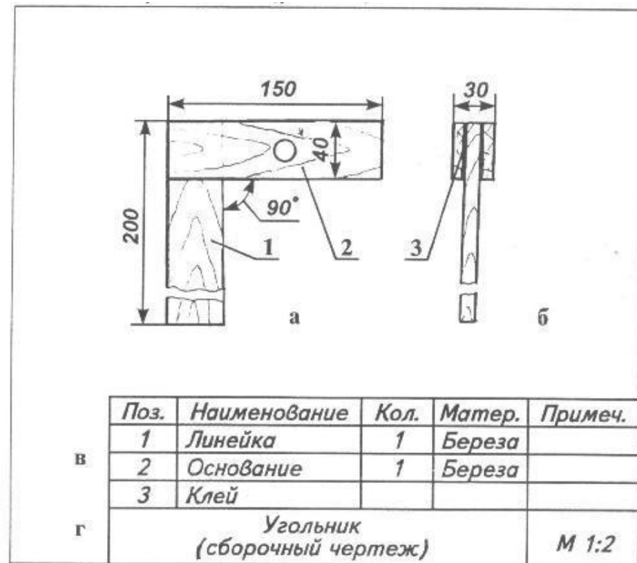
Рис. 1 . Сборочный чертеж угольника: а — главный вид; б — вид слева; в — спецификация; г — основная надпись
