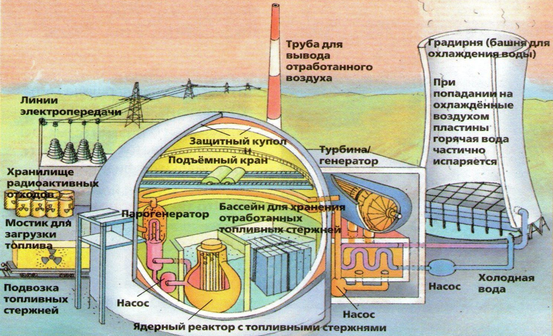
Схема атомной электростанции
