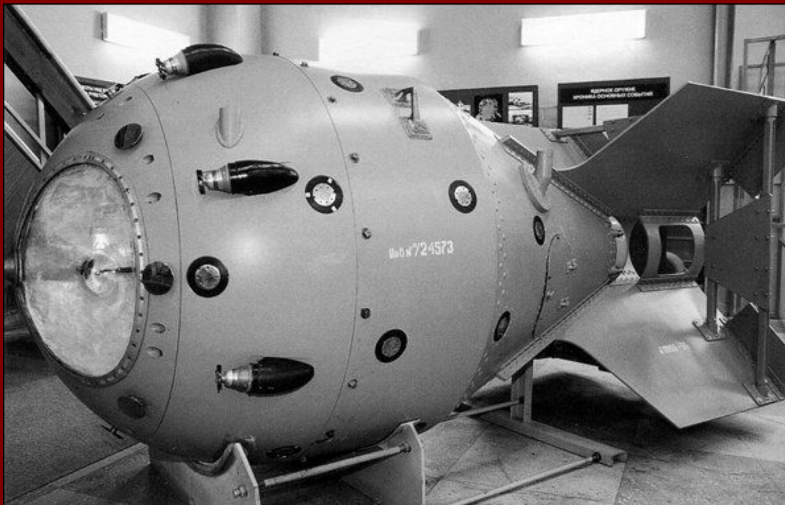
Водородная бомба
