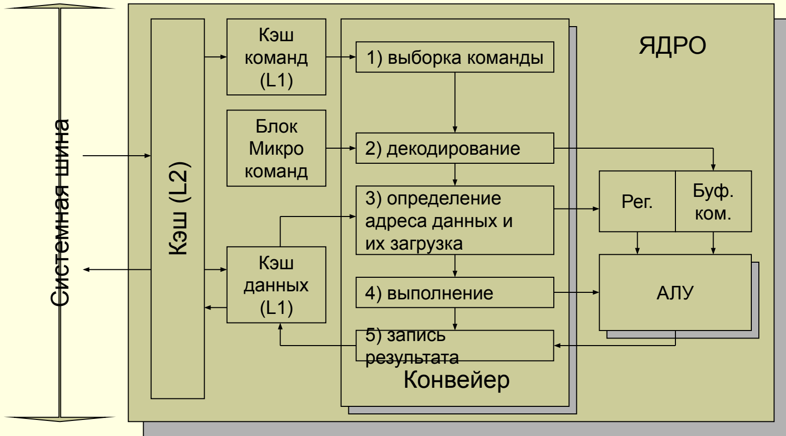
Структура ЦП серии P6
