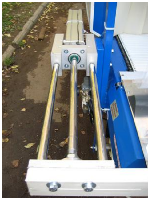
Пневмотолкатель группиратора
