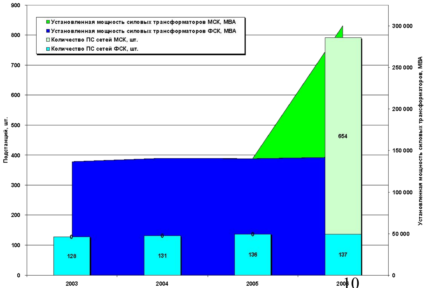
Динамика объема обслуживаемых ОАО "ФСК ЕЭС" подстанций, шт. / МВА
