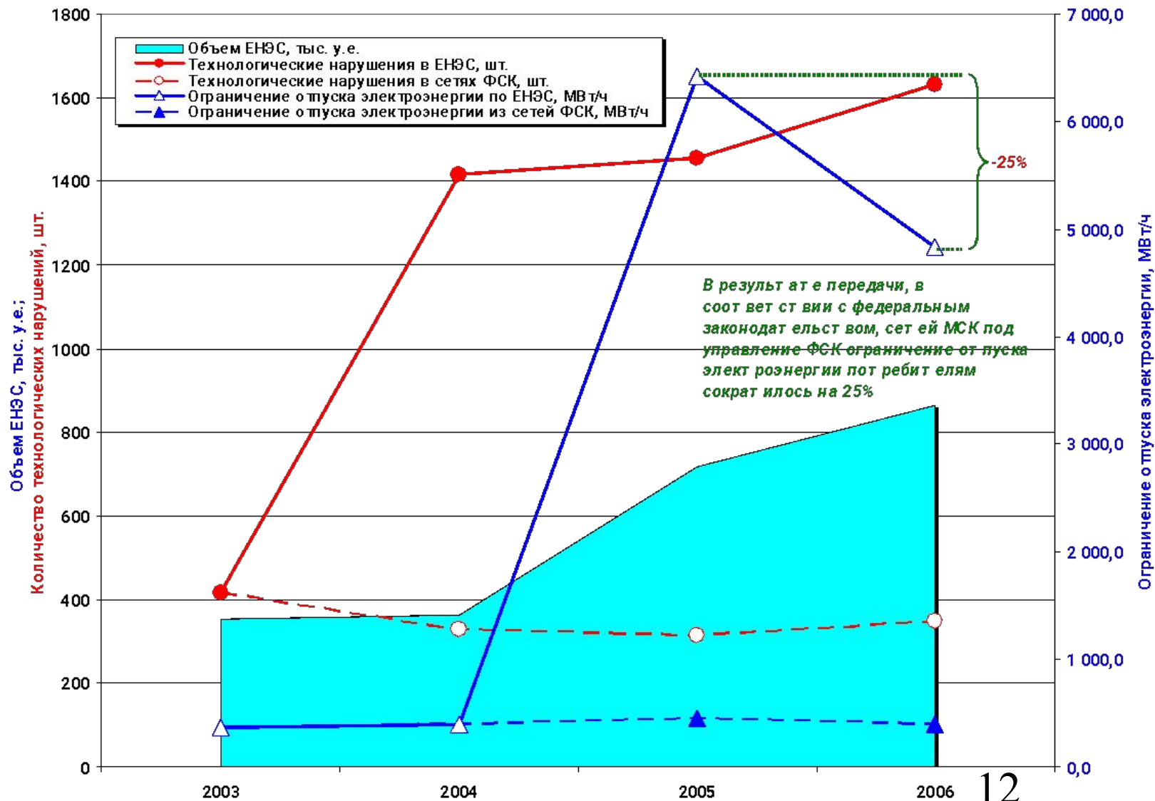
Динамика показателей ограничения отпуска электроэнергии и технологических нарушений
