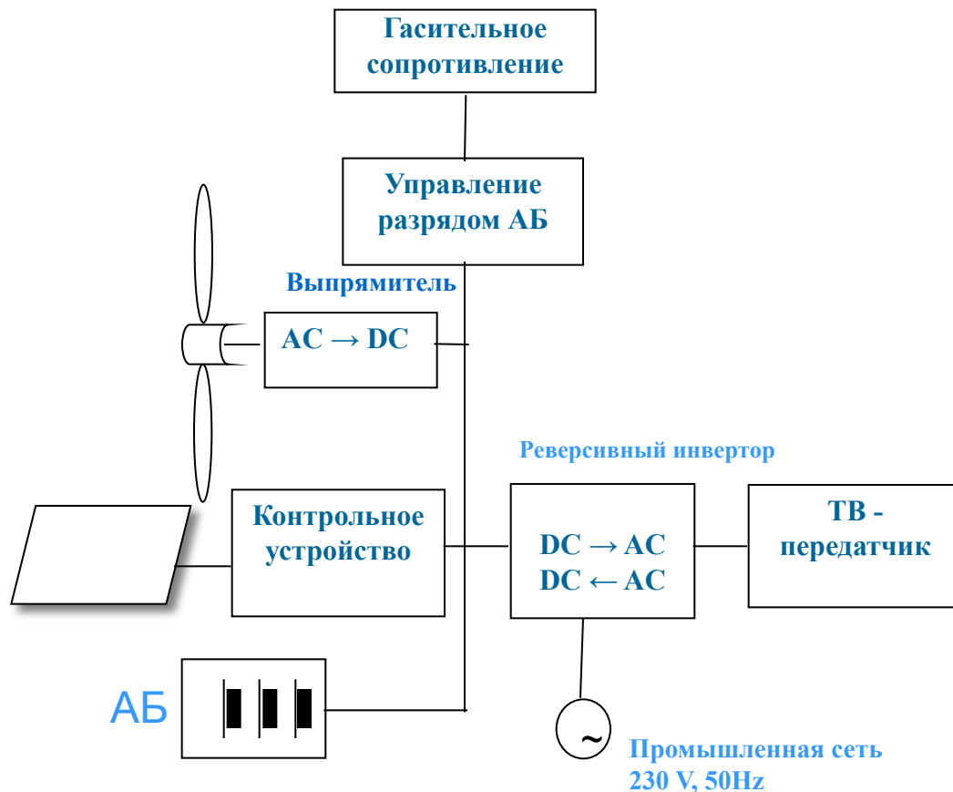
Рис.1. Структурная схема гибридного солнечно-ветрового источника электроэнергии
