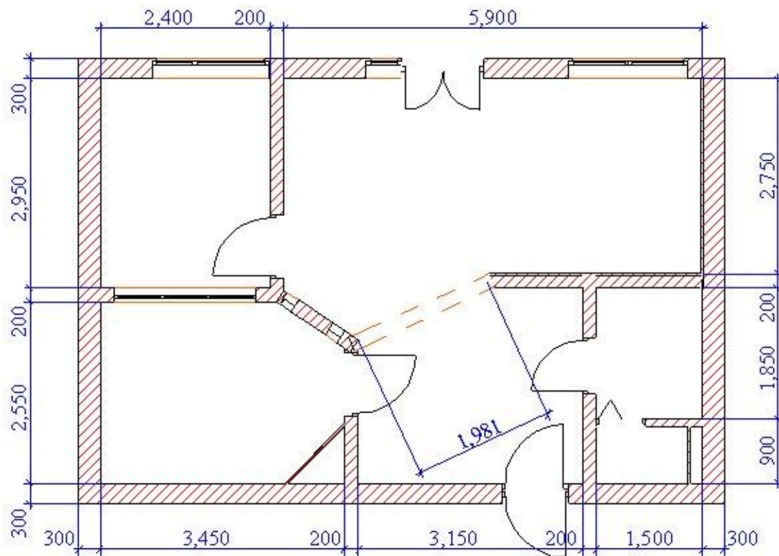
План двухкомнатной квартиры после перепланировки
