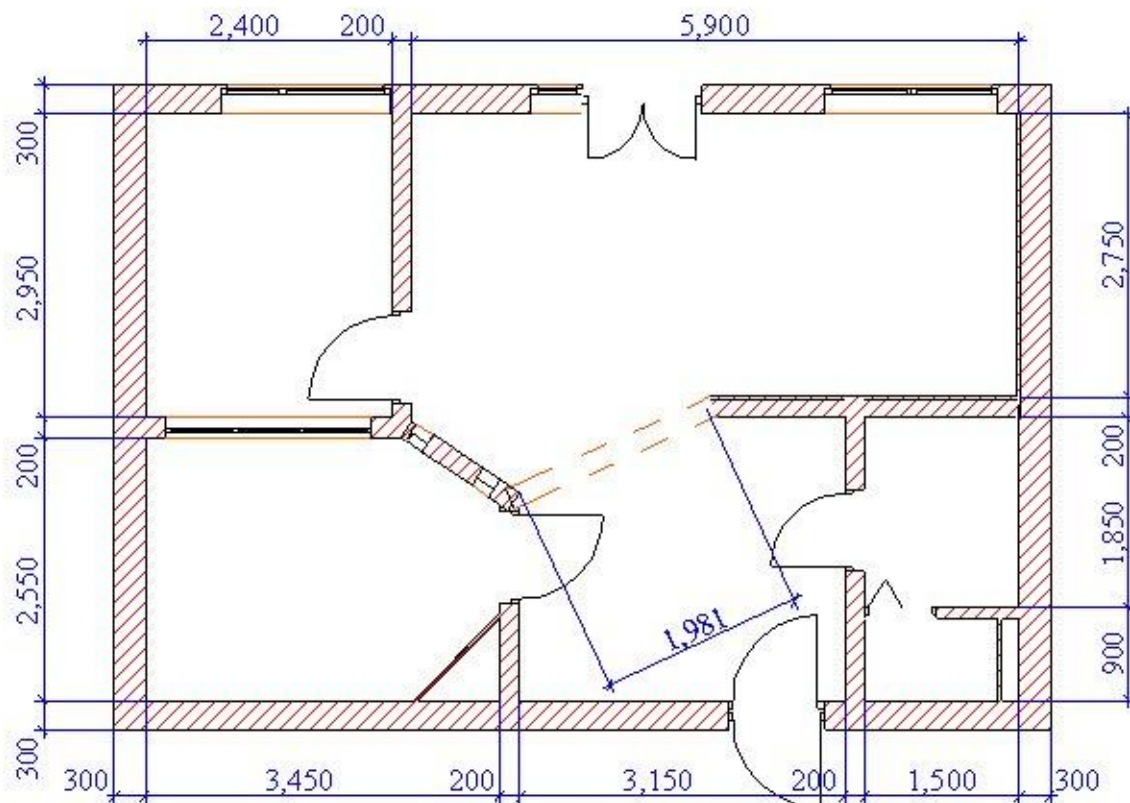
План двухкомнатной квартиры после перепланировки
