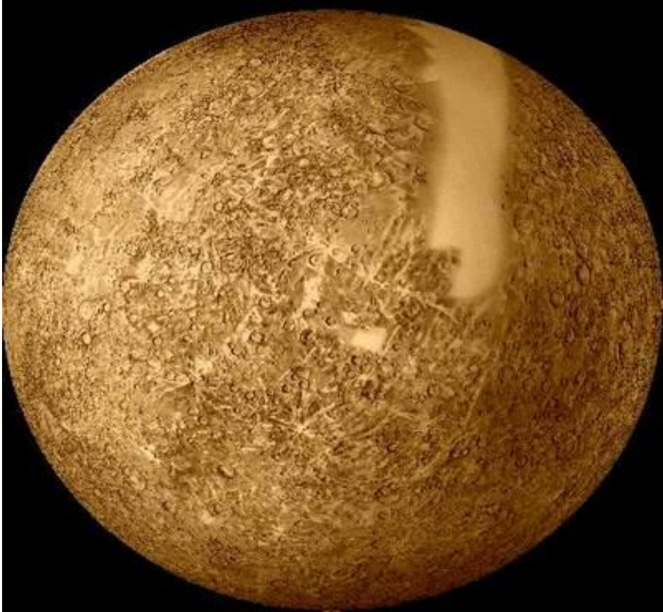
меркурий
