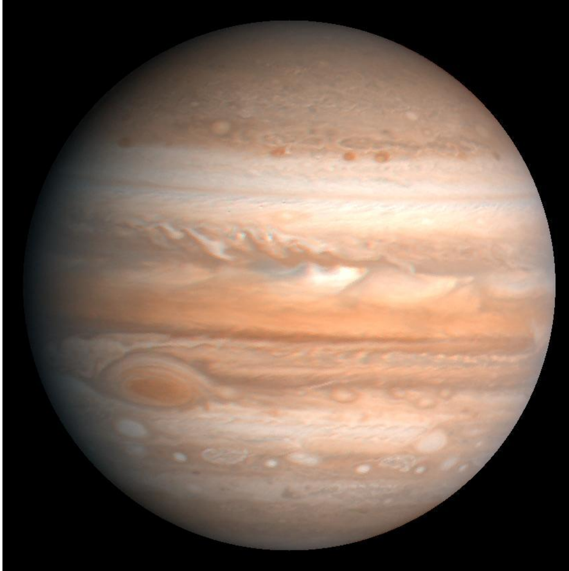
Юпитер
