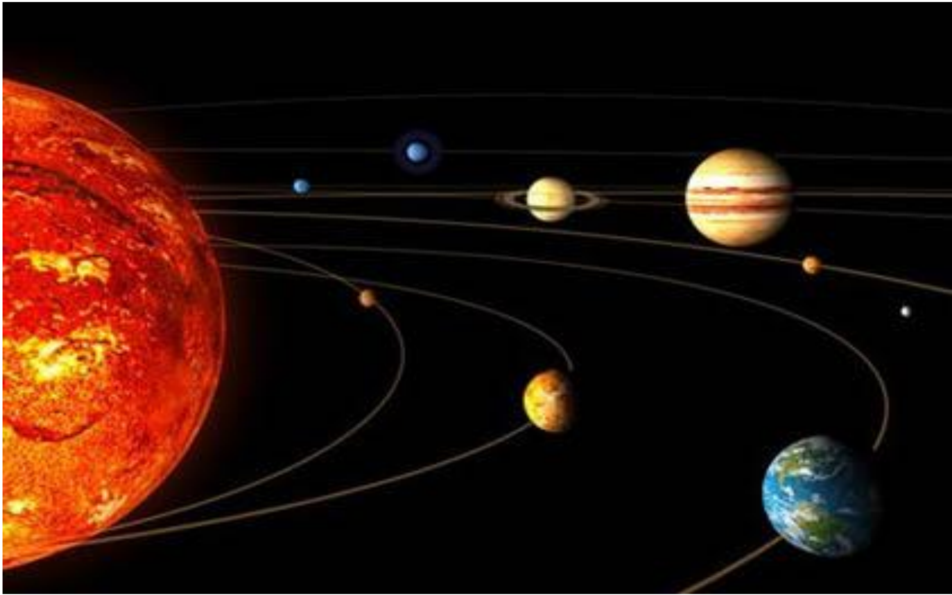
Солнечная система
