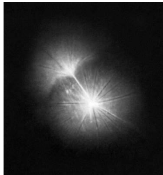
Фигуры Георга Кристофа Лихтенберга
