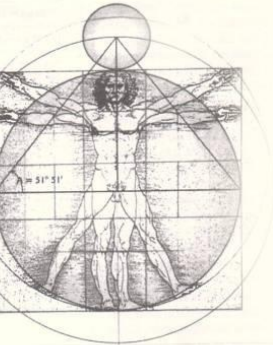
Рис. 9.39. Пропорции Земля—Луна.
