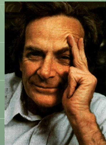
Ричард Фейнман (1918-1988)
