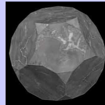
Усеченный додекаэдр
