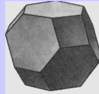
Усеченный октаэдр
